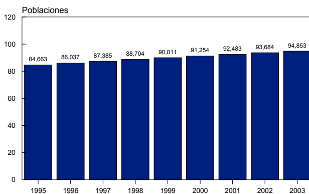
Comportamiento poblacional 1995 - 2003 Ipiales
