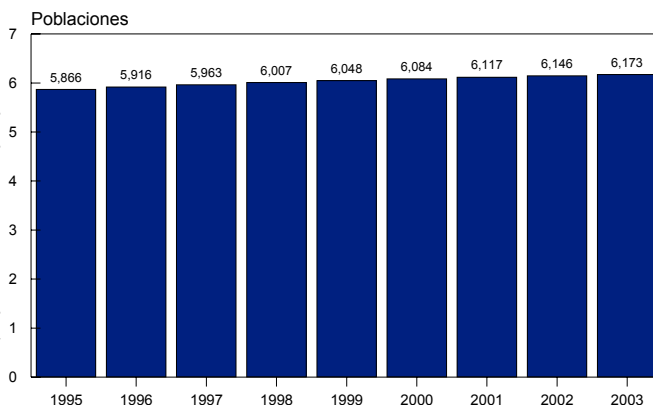
Comportamiento poblacional 1995 - 2003 Gualmatan
