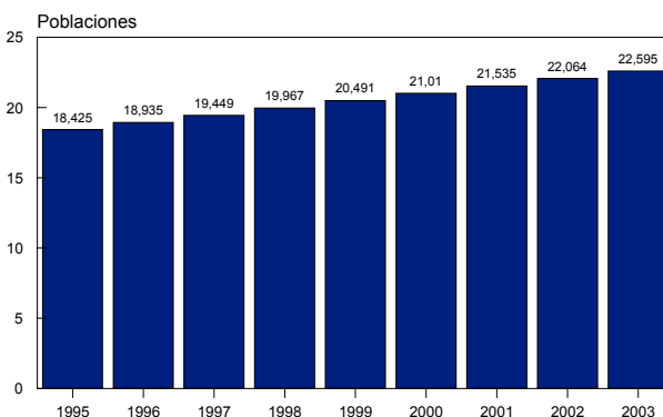
Comportamiento poblacional 1995 - 2003 Pupiales
