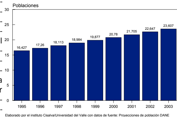
Comportamiento poblacional 1995 - 2003 Potosi
