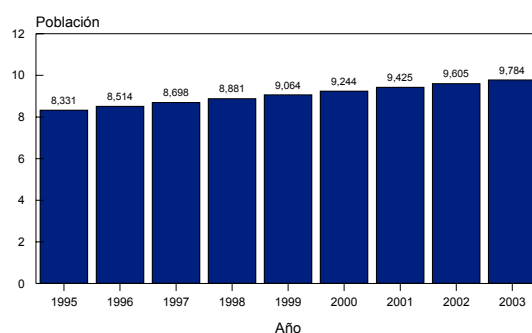
Comportamiento poblacional 1995 - 2003 Aldana
