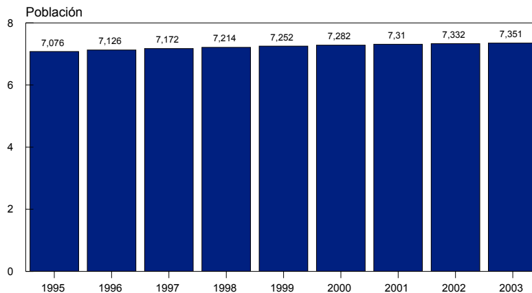
Comportamiento poblacional 1995 - 2003 Iles
